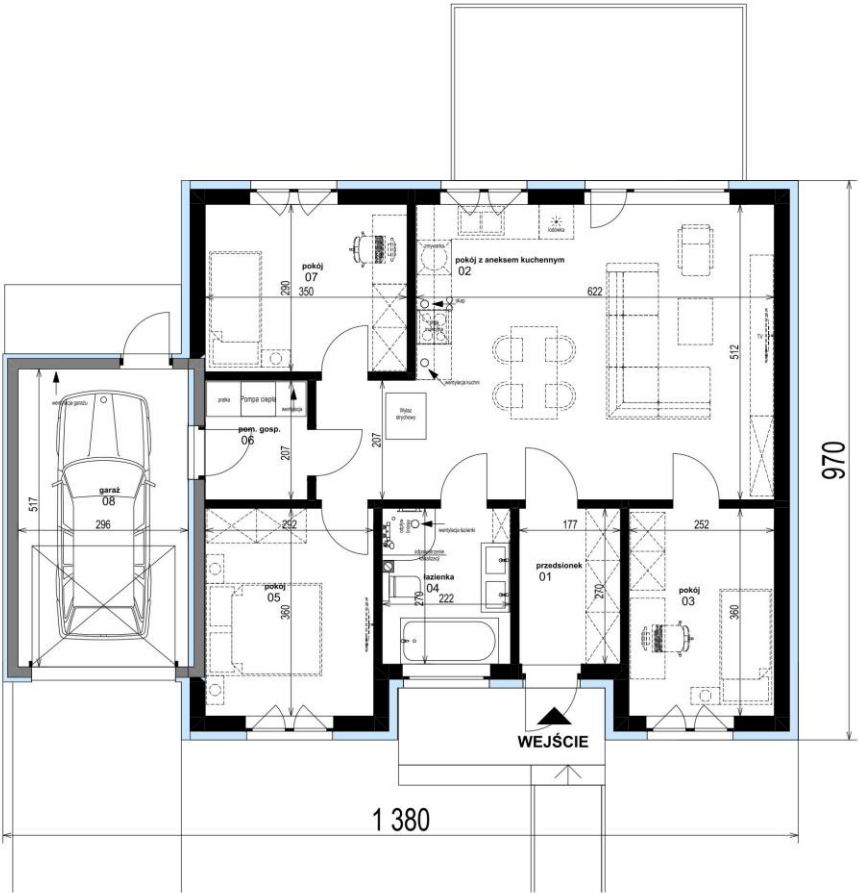
RZUT BUDYNKU
