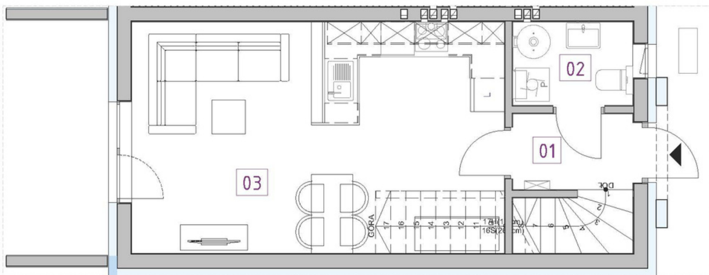
RZUT PARTERU
