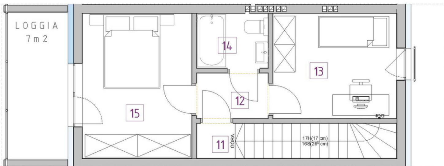
RZUT PIĘTRA
